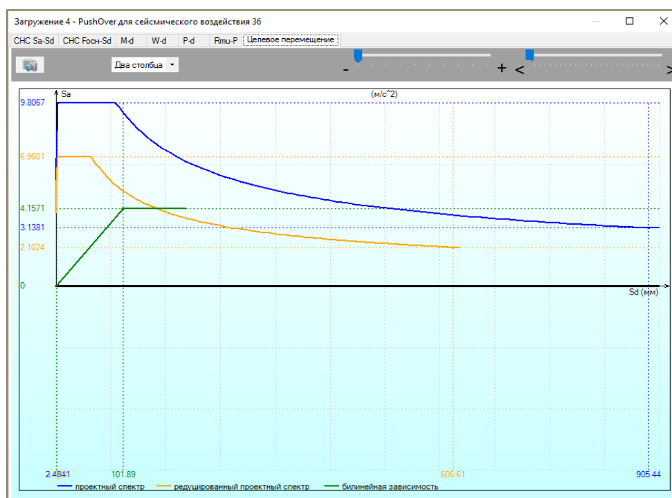
Рис. 12.6. Результаты по Pushover для 36-го модуля
